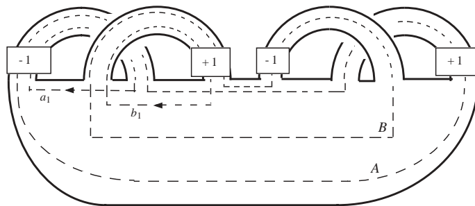
K' = J\# - J
